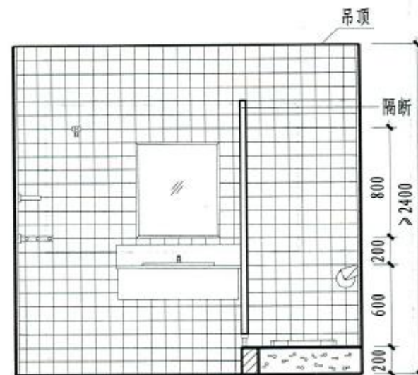
1-1 剖面
