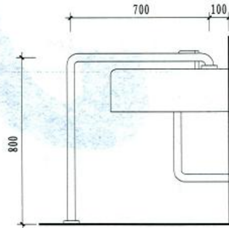
侧立面
