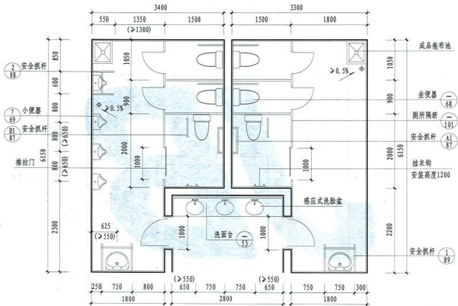
平面
