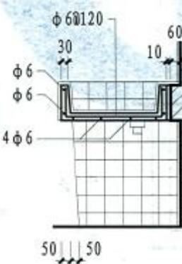
2-2剖面
