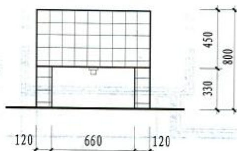
立面
