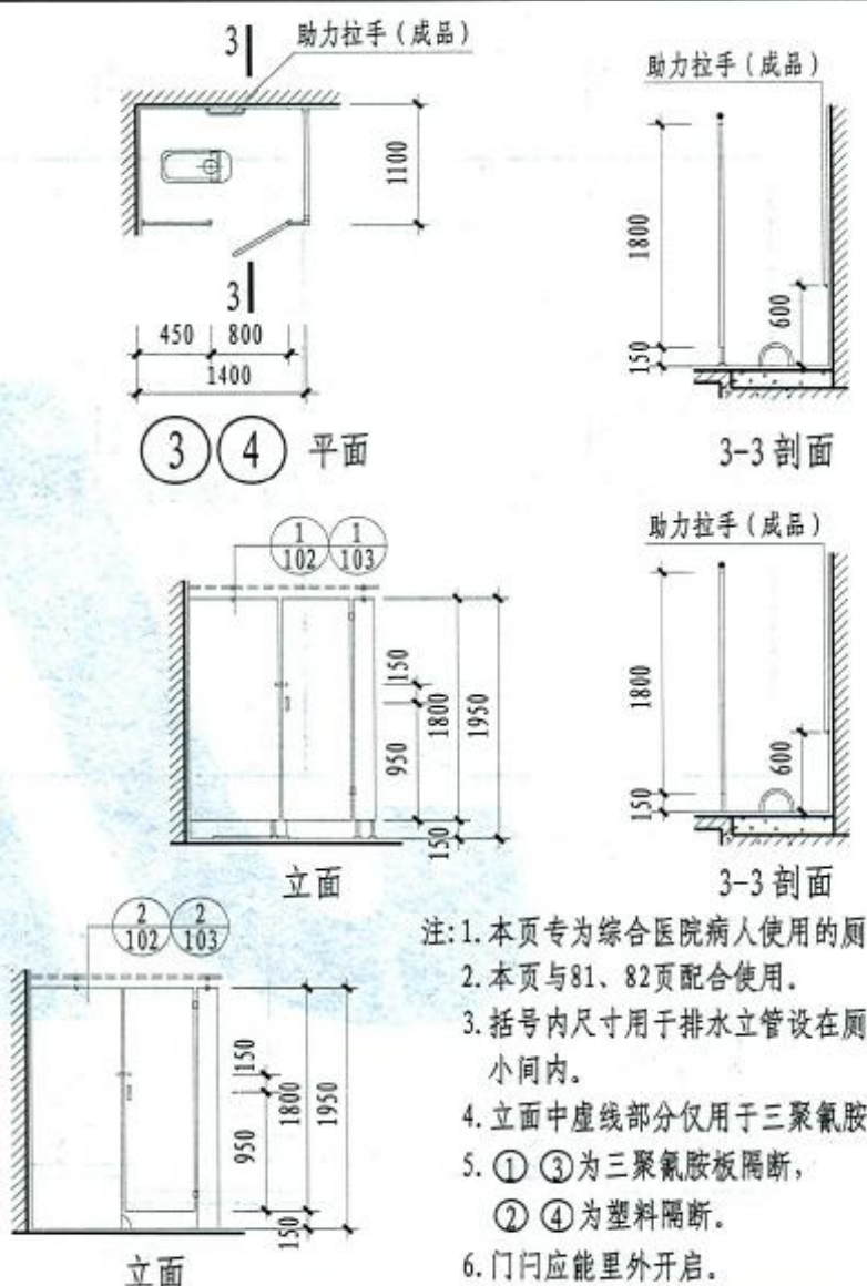
医院厕所隔断详图
