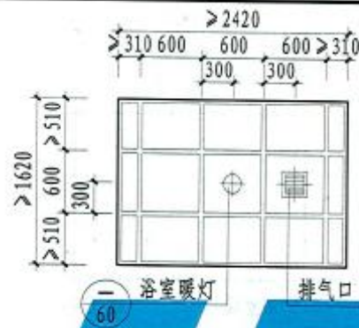
用于2型客房卫生间 ② ⑦
