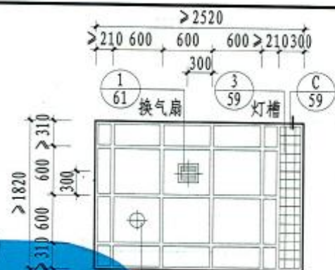
用于3型客房卫生间 ③ ⑧
