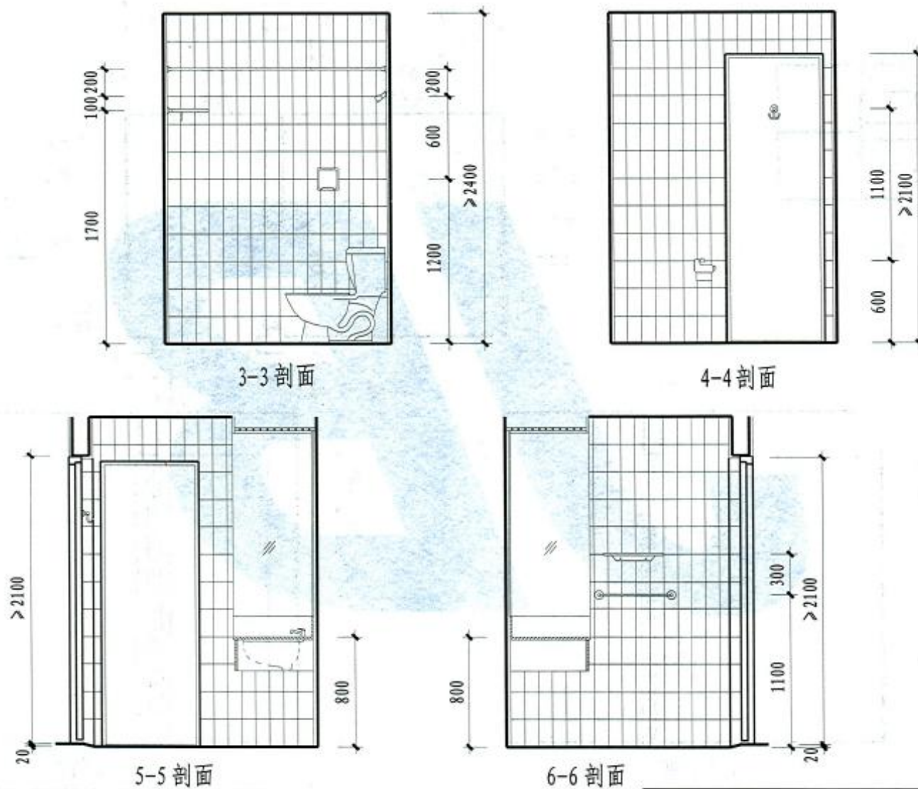
6型学生公寓卫生间(二)
