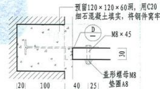
靠墙连接
