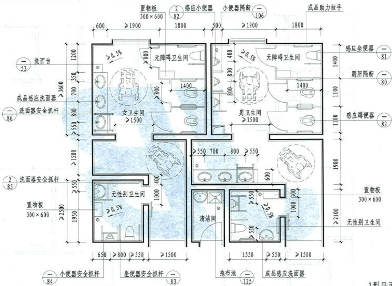
1型平面
