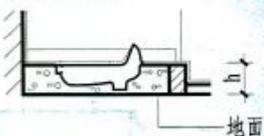
1-1剖面 (按普通型蹲便器绘制)
