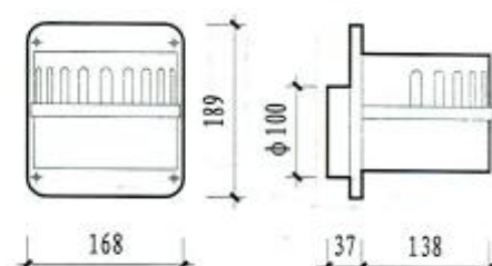
换气扇(成品)
