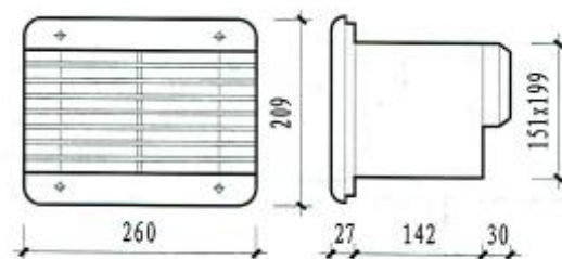
换气扇(成品)
