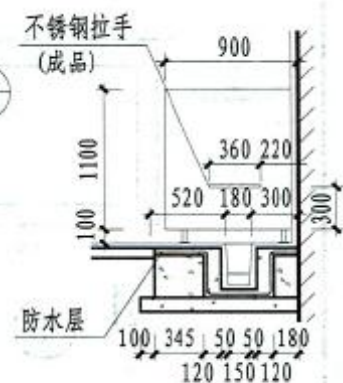
2-2剖面(用于地面)
