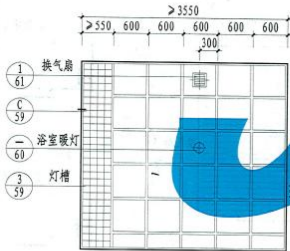
用于5型客房卫生间 ④ ⑨
