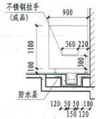
3a-3a剖面(用于楼层)
