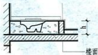
2-2剖面 (按连体型蹲便器绘制)
