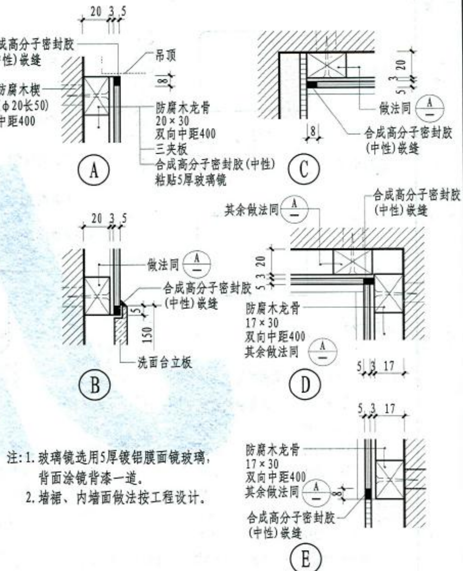
梳妆镜详图(三)
