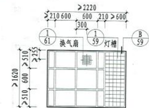
用于1型客房卫生间 ① ⑥
