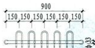
立面
